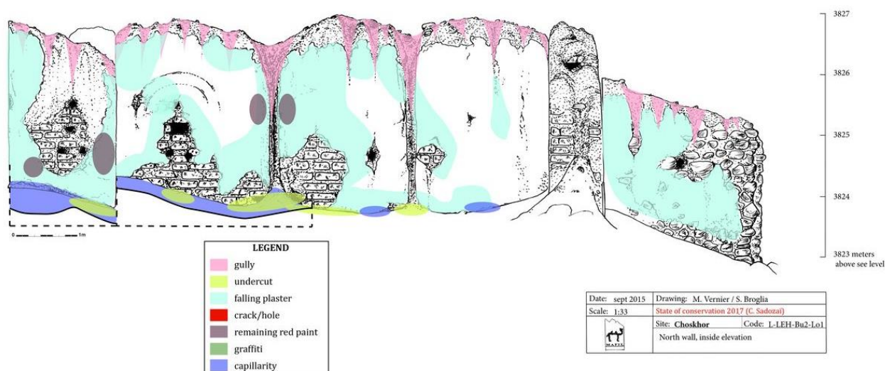
Mise en évidence des pathologies, façade interne du mur nord du temple 1, site de Leh Choskor, 2017. ©MAFIL_Sadozai / Vernier
